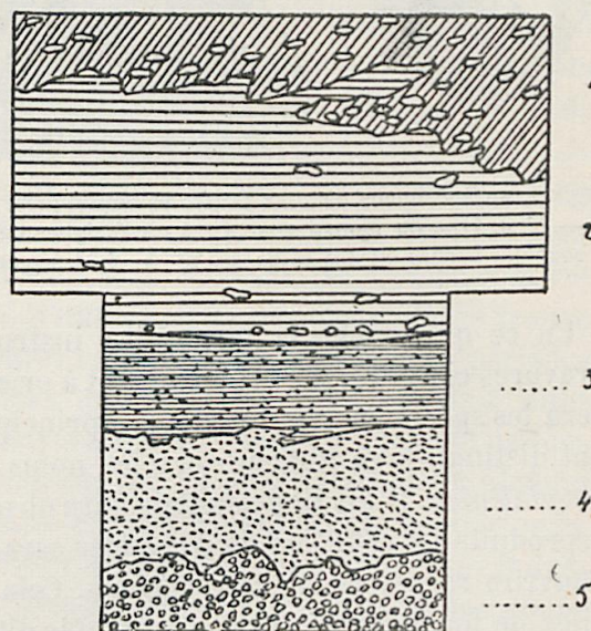
Fig. 15. — Coupe des sablières de la Somme.
