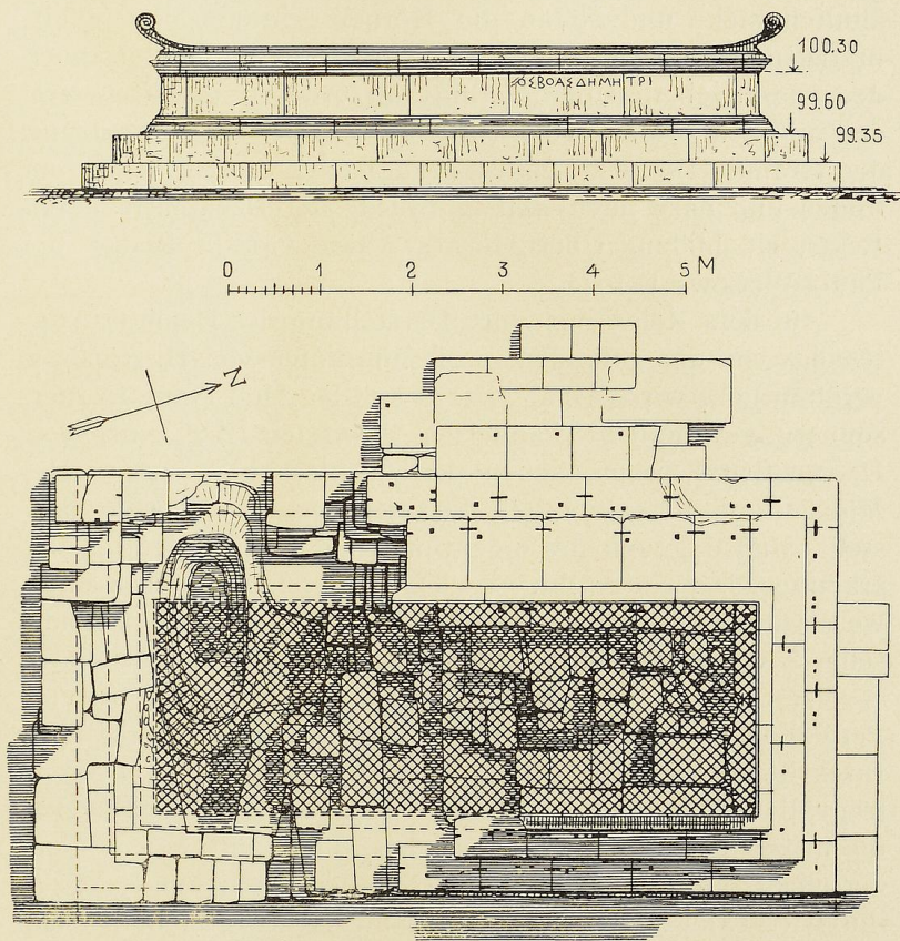
Abb. 7. Grundriss und ergänzter Aufriss des grossen Altars der Demeter.
