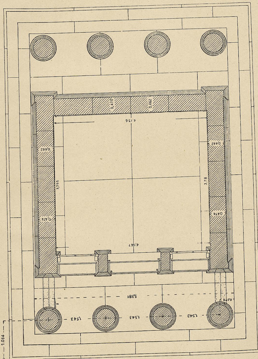
HORIZONTALER SCHNITT DES NIKETEMPELS IN DER HÖHE DER ORTHOSTATEN
