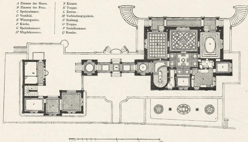
Grundriss zur Villa Patumbah des Herrn Grob-Zundel in Riesbach bei Zürich; erbaut von Chiodera & Tschudy, Architekten in Zürich.
