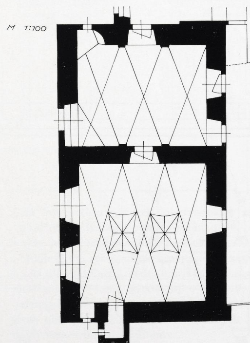
24. Kremnica, neskorogotický meštiansky dom č. 36, okolo roku 1520, časť pôdorysu a rez
