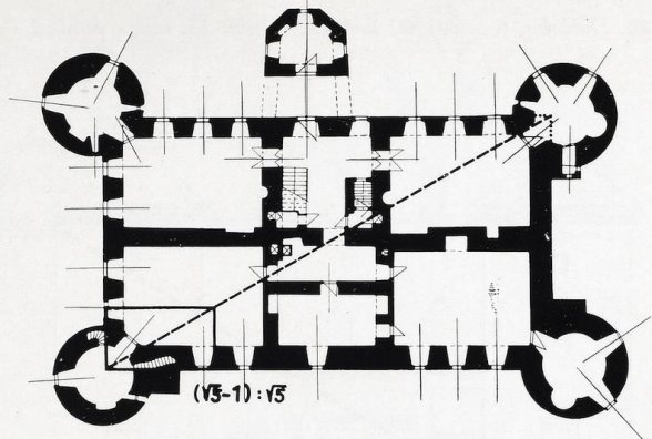
36. Markušovce, kaštieľ, koniec 16. stor., pôdorys
