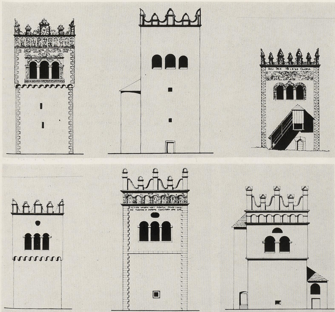
35. Spišské zvonice — Kežmarok 1586; Spišská Belá 1598; Strážky 1629; Vrbov 1644; Poprad 1658; Podolínec 1659. Všetky nárysy v rovnakej mierke 1:300
