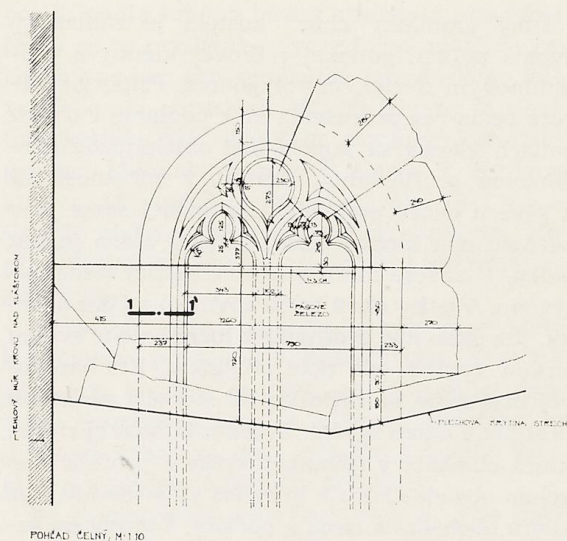
Časť gotického okna veže. Kresba M. Pichová
