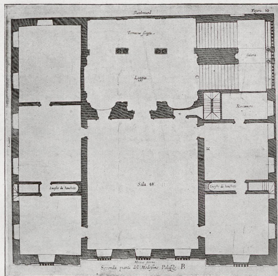
F. g. 7. — Genova: Villa Cambiaso - Pianta del piano nobile (dal Rubens).
