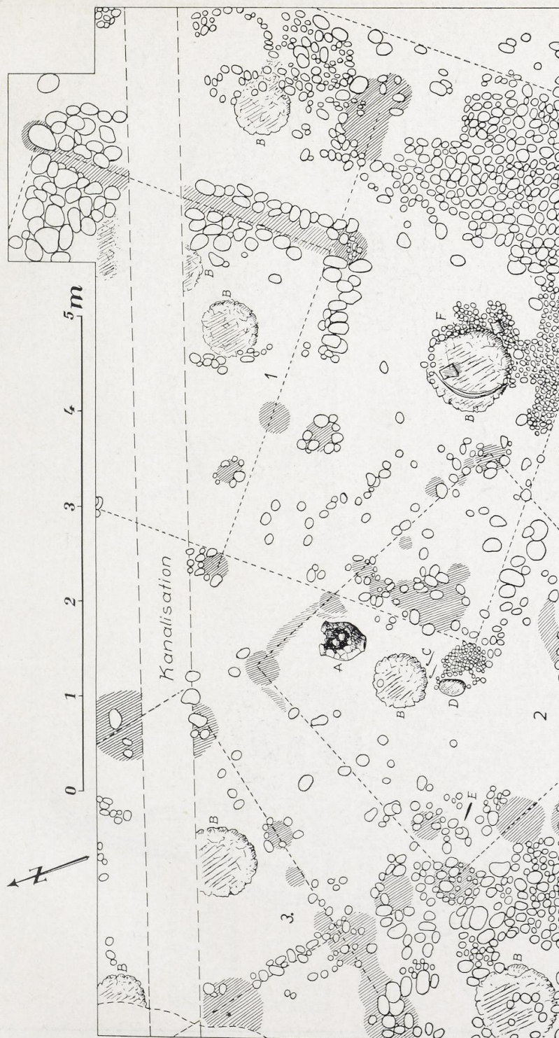
Säckingen, Schloßpark/Golfplatz. Schnitt 2 u. Flächengrabung: Hüttengrundrisse. A. Vorratsgefäß — B. Feuerstellen — C. Zwei Rollenkopfnadeln — D. Mahlstein — E. Bronze- meißel — F. Feuerbockreste
