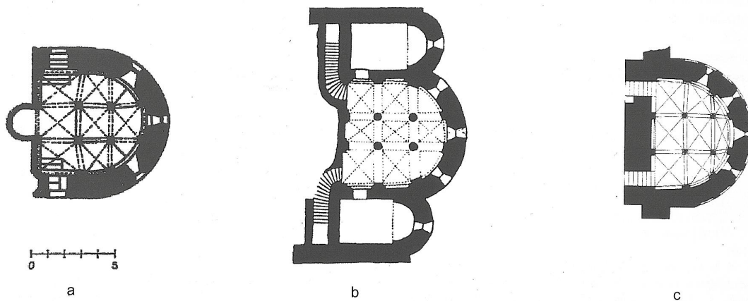
5. Krypty czteropodporowe: a – kościół Św. Maurycego w Amsoldingen, b – kościół Św. Maurycego w Aime, c – kościół Św. Wincentego w Galliano
