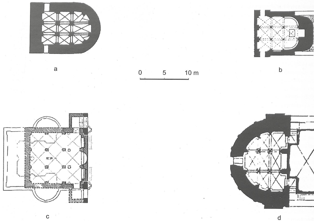
4. Nadmozańskie i nadreńskie krypty czteropodporowe: a – kościół Św. Hadelina w Celles, b – kościół Panny Marii w Hastière, c – kościół Św. Apostołów w Kolonii, d – katedra w Trewirze
