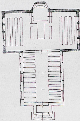
Dipl.-Architekt Otto Oskar Graebner, Berlin. Friedhofskapelle in Nauen. Um- und Erweiterungsbau. Der neue Teil ist im Grundriß schraffiert.
