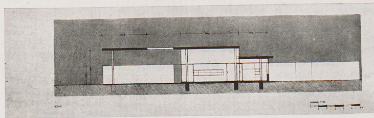
ARCHITEKT MARCEL BREUER. »HAUS FÜR EINEN SPORTSMANN«. GRUNDRISS, LAGEPLAN UND SCHNITT
