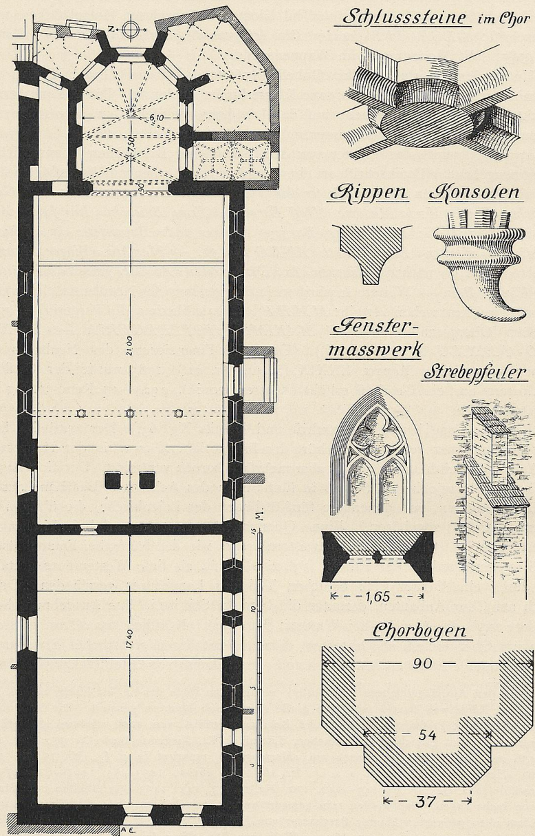
Fig. 63. Niederviehbach. Grundriß und Details der Klosterkirche.
