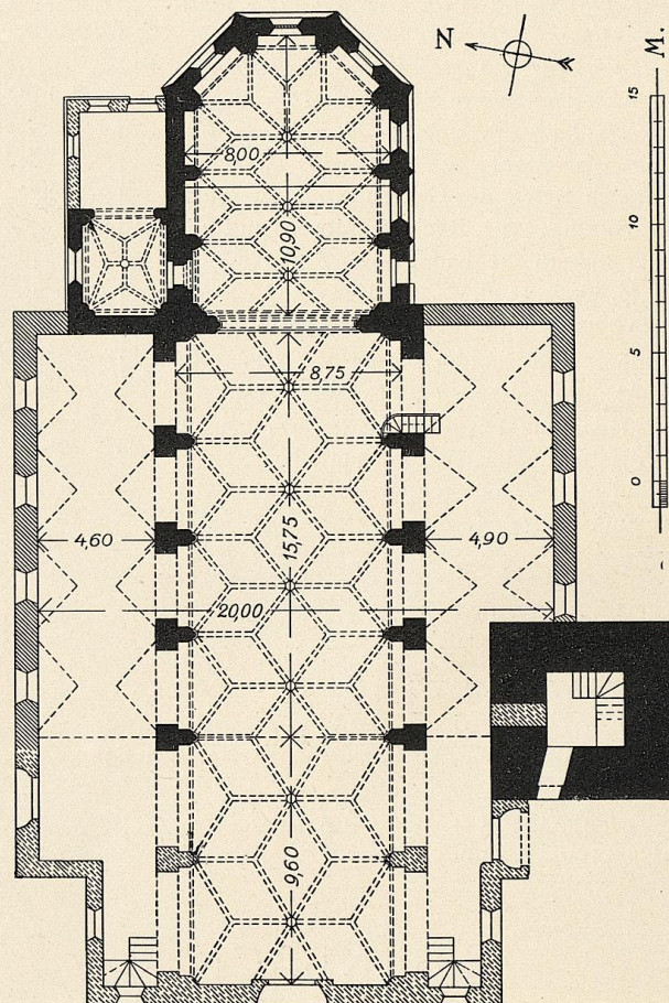
Fig. 67. Essenbach. Kirche. Grundriß.
