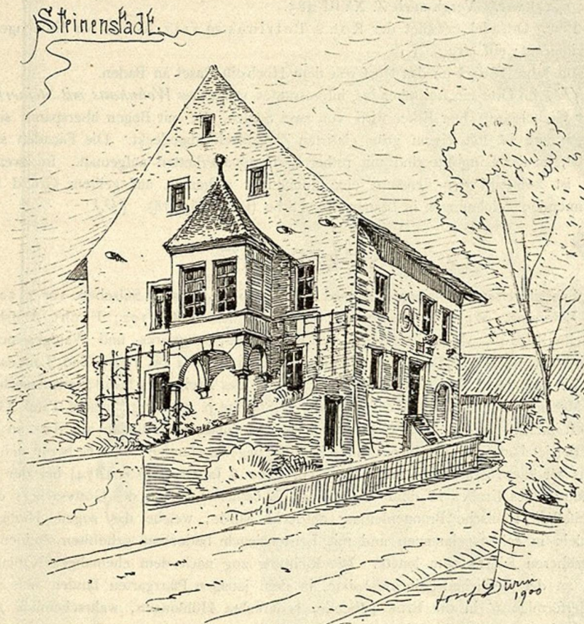
Fig. 78. Steinensstadt. Wohnhaus.
