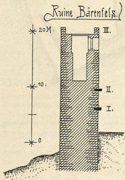
Fig. 111. Bärenfels. Vertikalschnitt des Rundturms.
