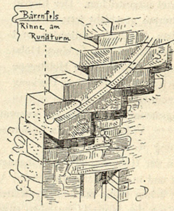
Fig. 112. Bärenfels. Rinne am Rundturm.
