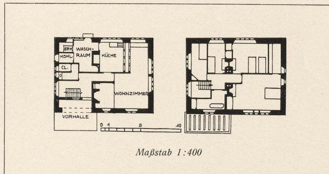
C. F. A. VOYSEY, LONDON Das Landhaus „Littleholme“ zu Kendal. — Ansicht und Grundrisse
