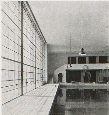
Schwimmbad · Piscine communale · Swimming-baths, Frankfurt am Main-Fechenheim. Architekt: Martin Elsaesser. Foto: Leistikow. Cf. Ausführliche Veröffentlichung · publication détaillée · detailed account: Das städtische Hallenschwimmbad in Frankfurt am Main-Fechenheim, herausgegeben von der städtischen Bäderdirektion
