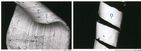
13. Fragmenty nici z opłotem metalowym z identycznej tkaniny broszowanej, jak w partiach boków ornatu 12: a) fragment opłotu nici metalowej; b) fragment nici z opłotem metalowym. Fotografie wykonane za pomocą mikroskopu elektronowego typu JOEL JSM-6380LA. Fot. M. Wróbel. Fragments of threads with metal foil from an identical brocaded fabric as in the sides of the chasuble: a) fragment of metallic thread foil; b) fragment of a thread with metal foil. Photographs taken with a JOEL JSM-6380LA electronic microscope. Photo: M. Wróbel.
