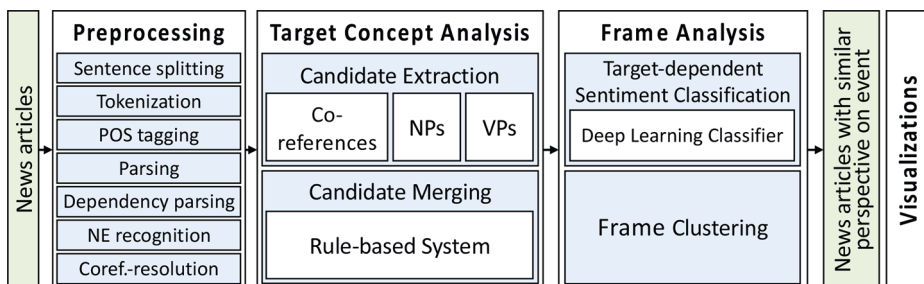
Abb. 1: Abfolge der einzelnen NLP-Schritte in der automatischen Identifikation von Media Bias. Die einzelnen Schritte werden von links nach rechts und von oben nach unten ausgeführt.
