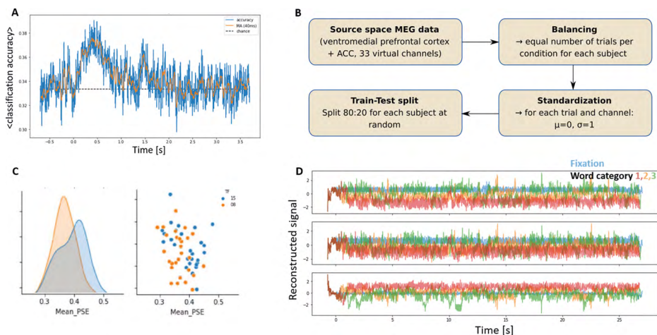
Abb. 2. A) Relative Akkuratheit der (out-of-sample) Klassifikation von 3 Aussagen-Typen auf der Basis von MEG-Zeitreihen ( y -Achse) in der Zeit ( x -Achse) gemittelt über N=28 Teilnehmer:innen. Zum Zeitpunkt 0 wird die jeweilige Aussage dargeboten. Etwa 400 ms nach Darbietung der Aussage ist die Dekodierfähigkeit am höchsten. B) Vorgehen zur Bestimmung von Hyperparametern der zur Analyse herangezogenen rekurrenten neuronalen Netze (RNNs). MEG-Daten aus dem präfrontalen Kortex werden extrahiert, die Anzahl der Trials wird pro Aussagen-Bedingung balanciert, die Daten werden dann standardisiert und in ein Trainings- und Testset eingeteilt (80 % Training, 20 % Test). RNNs werden dann an den Trainingsdaten trainiert und auf den Testdaten evaluiert. C) Vergleich der Abweichung (hier in Termen der Abweichung auf dem rekonstruierten Frequenzspektrum) zwischen beobachteten und durch die RNNs rekonstruierten MEG-Testset-Daten für zwei Einstellungen (farblich gekennzeichnet) des RNN-Modells. Der Vergleich zeigt, dass sich die Rekonstruktion verbessert, wenn wir ein kurzes ‚Teacher Forcing‘-Intervall wählen (hier nicht näher erläutert, cf. Brenner et al., accepted). D) Konkretes Beispiel von rekonstruierten MEG-Zeitreihen. Die RNN-Modelle werden nach initialer Auslenkung durch ein Fixationskreuz (blau) oder drei Wörter unterschiedlichen Selbstbezugs (rot, orange, grün) für 25 Sekunden laufen gelassen. Die rekonstruierten Zeitreihen zeigen teilweise unterschiedliches Verhalten als Antwort auf die unterschiedlichen Reize.
